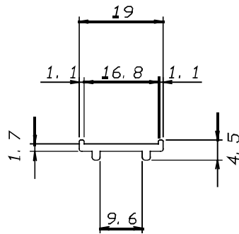
拡大図 \phi=1/1
