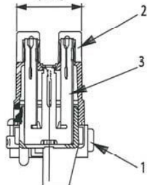
断面図 A-A
